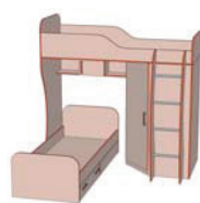
Вариант №3 2040x2040x2070
