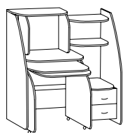
ИД 01.152 Стол компьютерный Г586-1010xШ1200xВ1242
